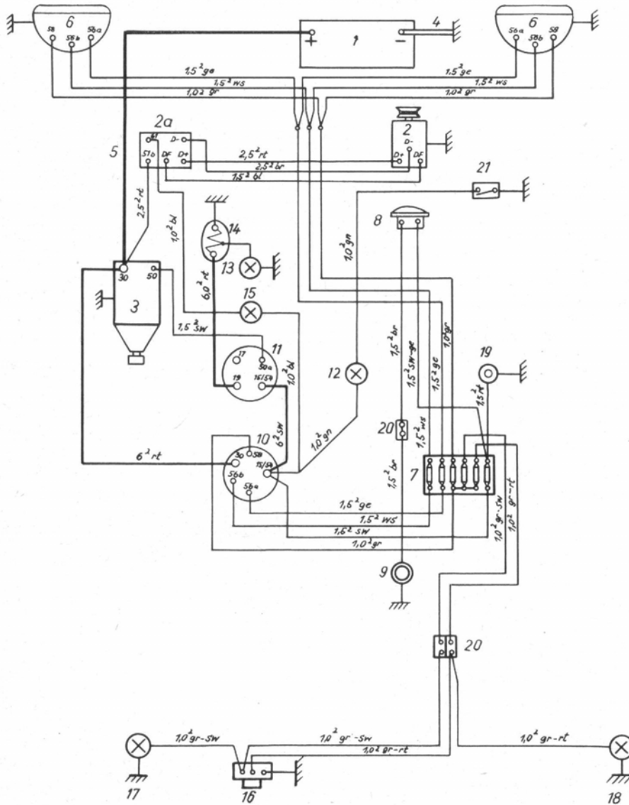
Bild 35 Schaltschema
